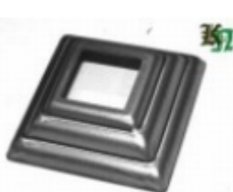
Основание баясины, арт. 13.326.01 57x57x1мм, кв.20x20мм Вес: 0.02 кг Цена: 20 руб.
