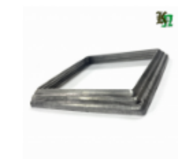
Основание блясины, арт. 13.310.02 122x122x1мм, кв.100x100мм Вес: 0.06 кг Цена (за шт): 50 руб.
