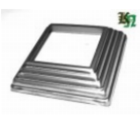
Основание блясины, арт. 13.310.01 142x142x1мм, кв.100x100мм Вес: 0.135 кг Цена: 70 руб.
