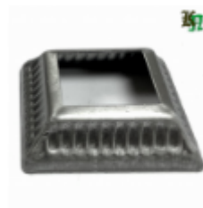
Основание блясины, арт. 8.6030 60x60x1мм, кв.30x30мм Вес: 0.04 кг Цена (за шт): 45 руб.
