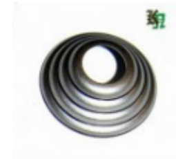
Основание баясины, арт. 13.348.01 д=50x1мм, отв.д=17мм Вес: 0.02 кг Цена: 11 руб.
