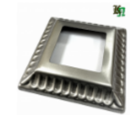
Основание блясины штампованное, арт. 8.881 170x170x1 кв. 80x80 Вес: 0.21 кг Цена (за шт): 150 руб.
