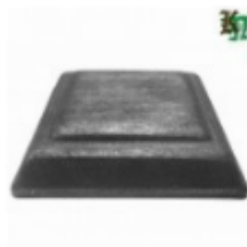
Основание балясины, арт. 7.310 100x100x20мм, без отв. Вес: 0.27 кг Цена: 90 руб.
