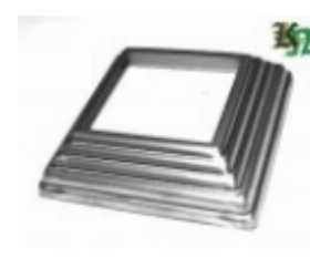
Основание блясины, арт. 13.380.01 122x122x1мм, кв.80x80мм Вес: 0.11 кг Цена: 50 руб.
