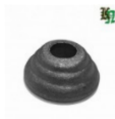
Основание блясины, арт. 7.346 д=40мм, отв.д=12мм Вес: 0.06 кг Цена: 52 руб.
