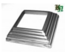
Основание блясины, арт. 13.360.01 108x108x1мм, кв.60x60мм Вес: 0.07 кг Цена: 40 руб.
