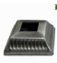
Основание баясины, арт. 8.6020 60x60x1мм, кв.20x20мм Вес: 0.04 кг Цена (за шт): 43 руб.
