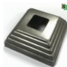
Основание баясины, арт. R10436.02 80x80x1мм, кв.25x25мм Вес: 0.075 кг Цена (за шт): 10 руб.
