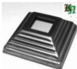
Основание баясины, арт. 10436.01 80x80x1мм, кв.25x25мм Вес: 0.075 кг Цена: 29 руб.
